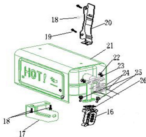
FIG.10 MUFFLER ASSY
